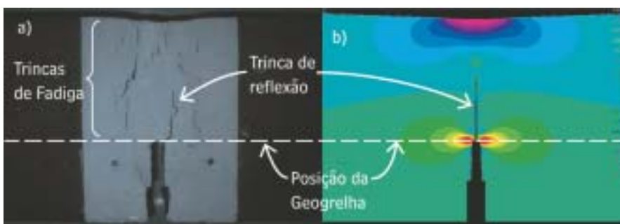
Figura 3 – (a) Padrão de trincamento nas vigas com geogrelha, após 500 mil ciclos de carga; (b) Simulação numérica
