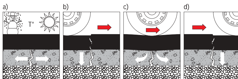
Figura 1 – Solicitações mecânicas em um pavimento trincado
